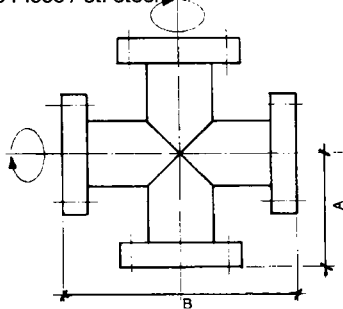
CF-Kreuzstück, 2 Flansche drehbar / Edelstahl Cross Piece / st. steel
