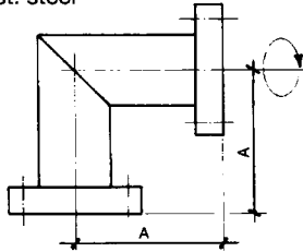
CF-Winkelstück, 1 Flansch drehbar / Edelstahl Elbow / st. steel
