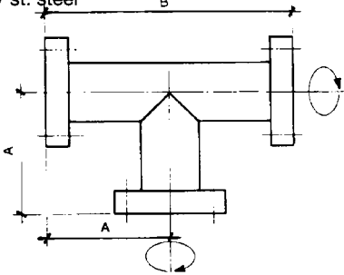
CF-T-Stück, 2 Flansche drehbar / Edelstahl Tee / st. steel
