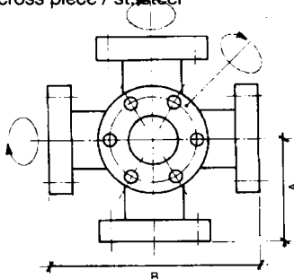
CF-Doppel-Kreuzstück, 3 Flansche drehb. / Edelst. 6 way cross piece / st. steel
